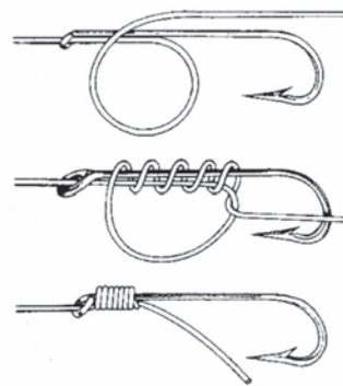
Snell Knot
